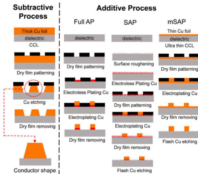
圖一：PCB 製程差異比較
